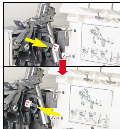
Unikátní navlékač levého chapače
