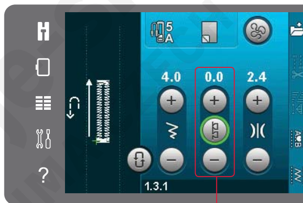
Vyvážení vpřed/vzad
